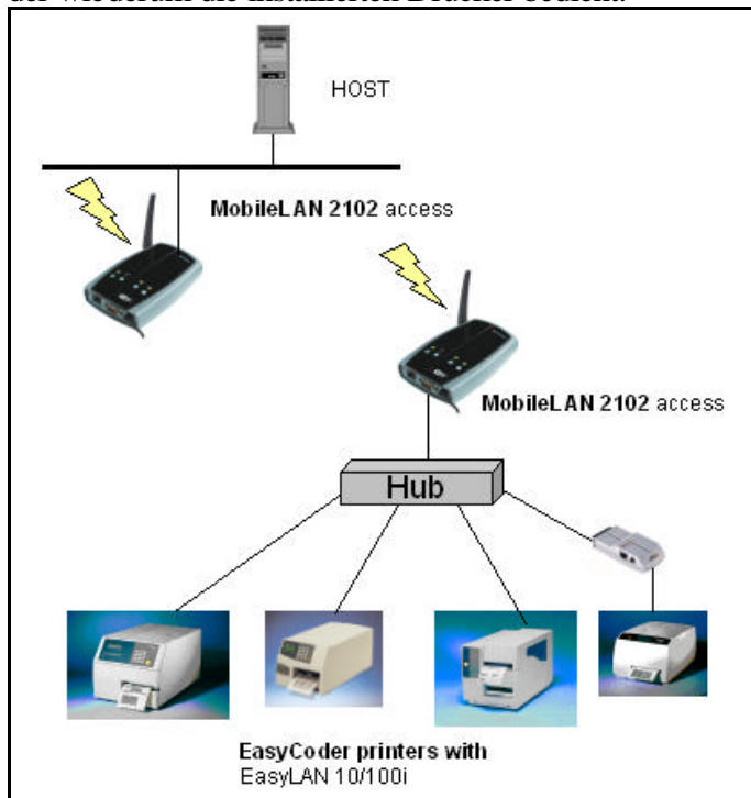
Abb. 2 – Anbindung mehrerer Drucker an ein WLAN mittels Hub
